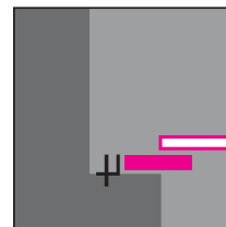
Bij montage van het kozijn gedeeltelijk in de dagopening (tot max. 50 mm per zijde) is een bevestiging naast het kozijn noodzakelijk.
